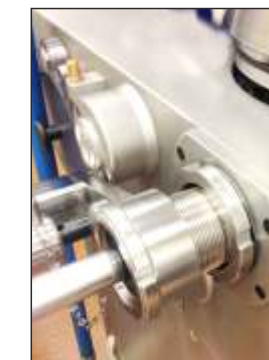
Füllrohrträger Handwerk Sortenwechsel mit minimalen Brätresten Stuffing horn support for small trade business Product changeover with minimal residues
